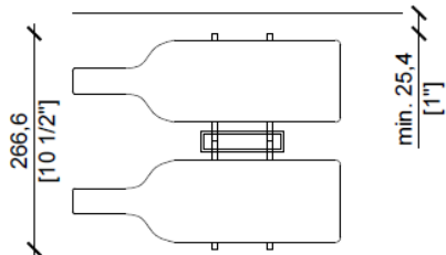
M1 - Magnum 1 Deep 2 Sides
