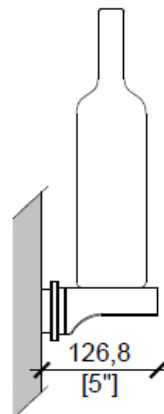
LS - Light Shelf
