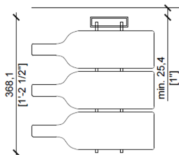
M3 - Magnum 3 Deep 1 Side
