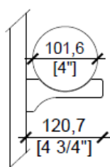
M1 - Magnum 1 Bottle
