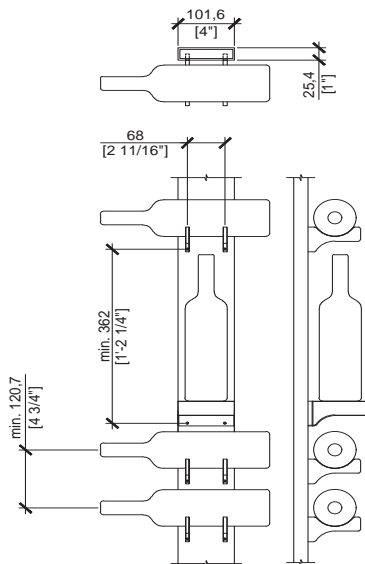
Post & Fin Detail
